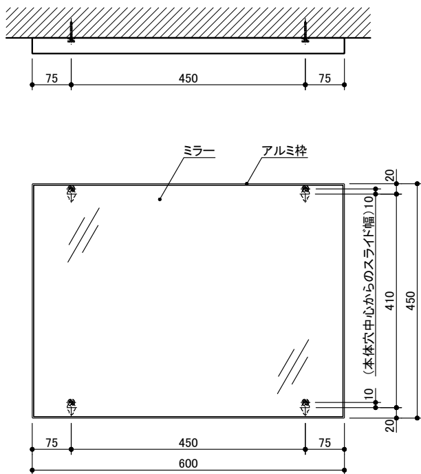
W600×H450 設置時
