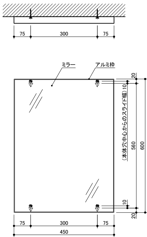
W450×H600 設置時
