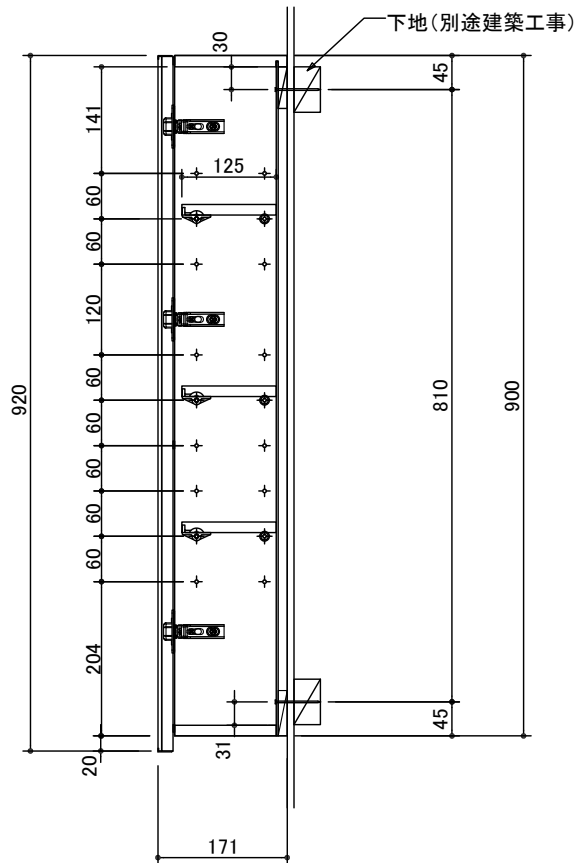
A 断面図
