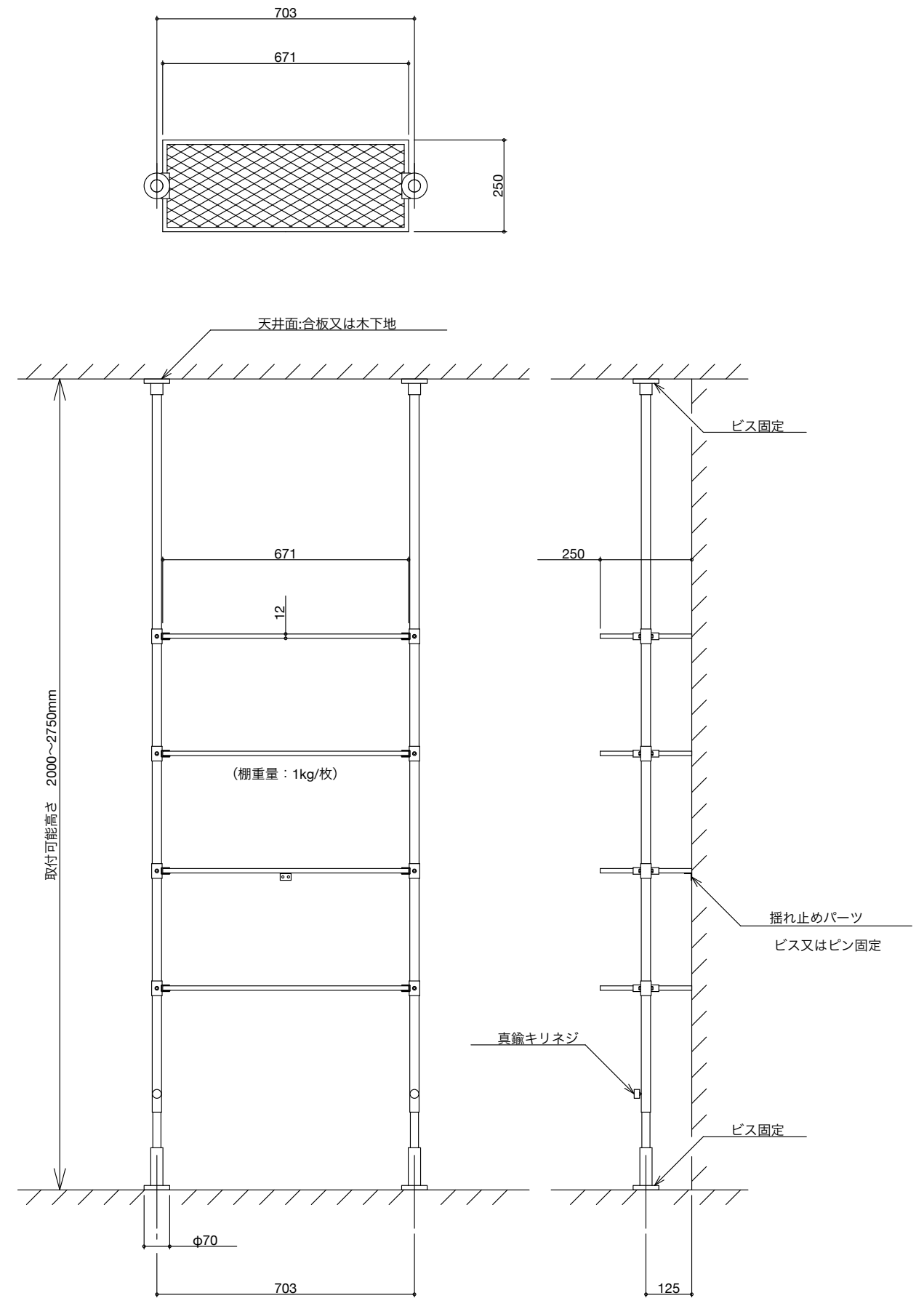
Rack A set 製品図
