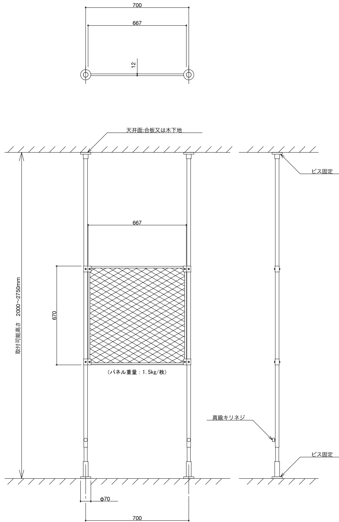
Partition A set 製品図
