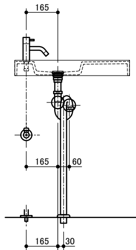
単水栓
