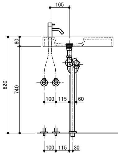
混合水栓
