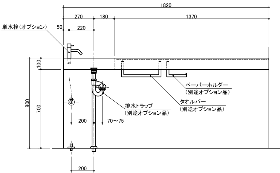
単水栓 給排水位置
