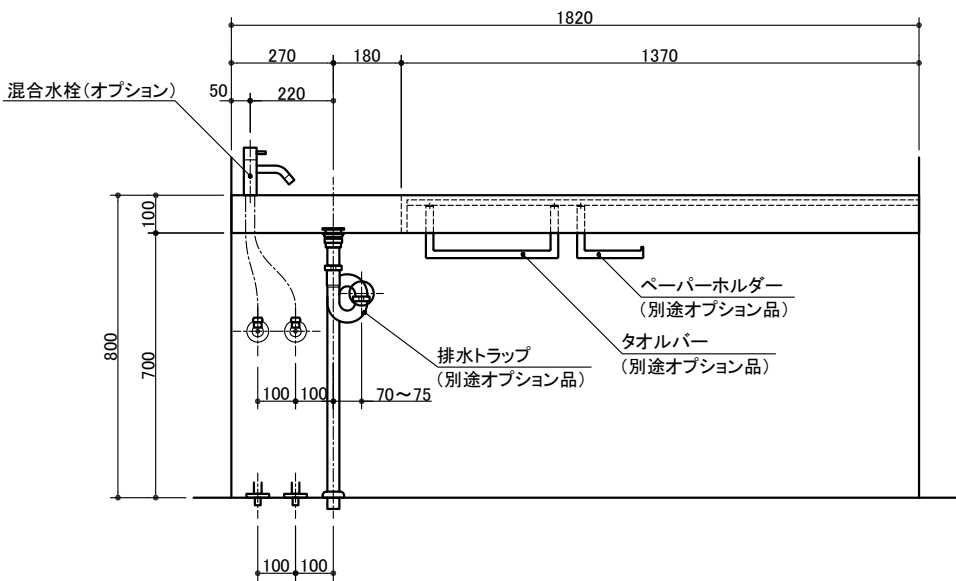
混合水栓 給排水位置
