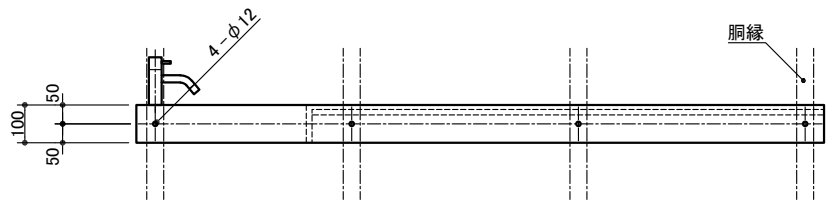
カウンター固定用アンカーボルト位置
