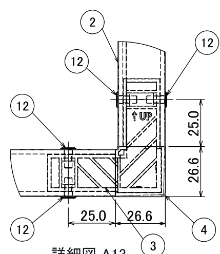
詳細図 A13 スケール 1 : 2
