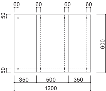
壁固定ネジ位置【W1200】
