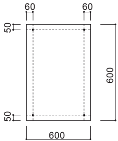
壁固定ネジ位置【W600】
