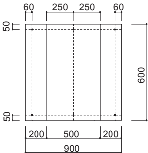
壁固定ネジ位置【W900】
