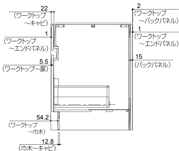
【バックパネル型 詳細納まり図】
