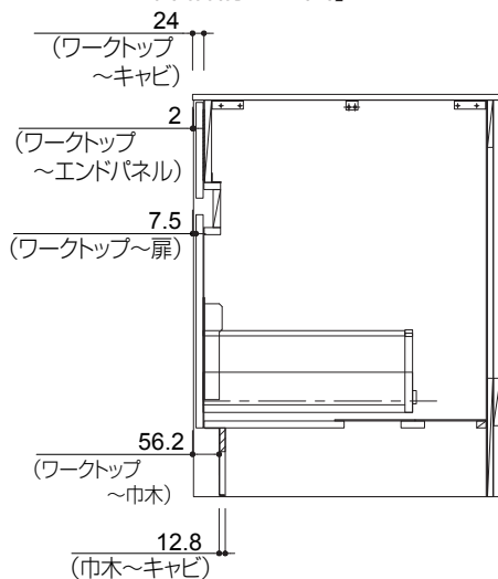
【ウォール型 詳細納まり図】
