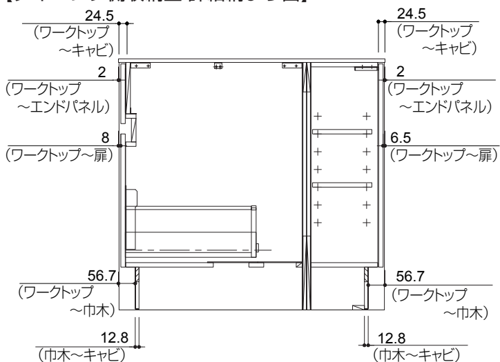
【ダイニング側収納型 詳細納まり図】
