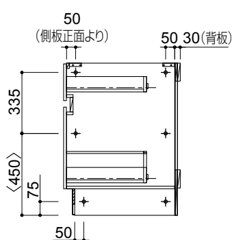
【ウォール型連結位置図】
