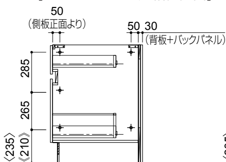
【バックパネル型連結位置図】
