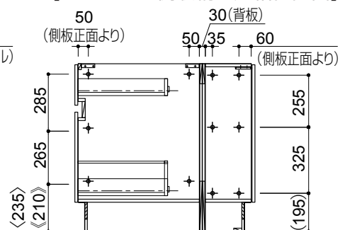
【ダイニング側収納型連結位置図】
