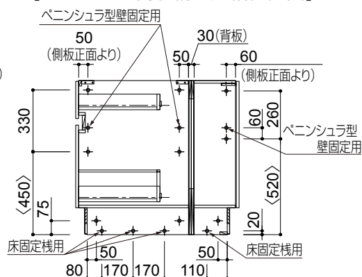
【ダイニング側収納型連結位置図】
