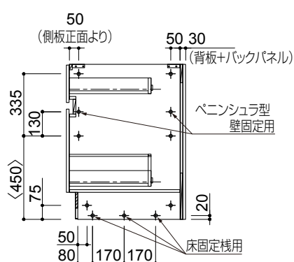
【バックパネル型連結位置図】
