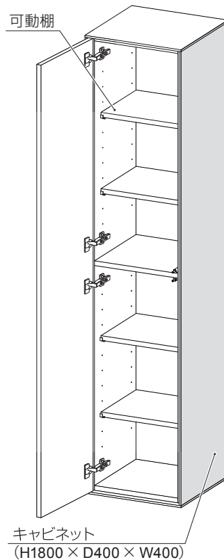
開き扉トールタイプ （1枚開き扉 H1800）
