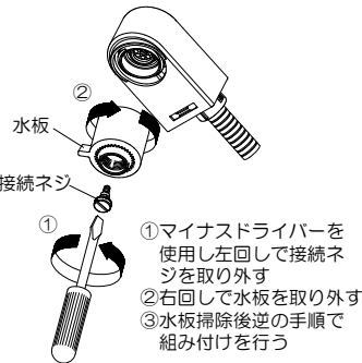
〈水板の取り外し方法〉
