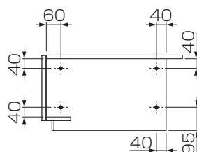
＜深型食洗キャビネット 側面図＞
