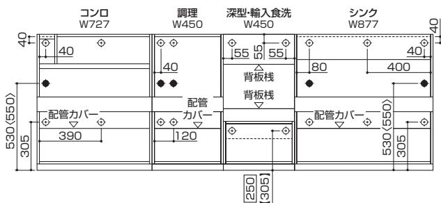
(ワークトップ W2550/深型食洗機・輸入食洗機(W450)設置の場合)
