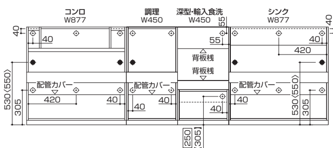
(ワークトップ W2700/深型食洗機・輸入食洗機(W450)設置の場合)
