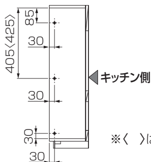
＜背面収納キャビネット 側面図＞
