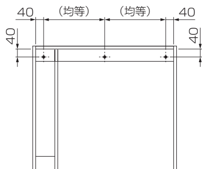
＜コンロ下ベースキャビネット 上面図＞
