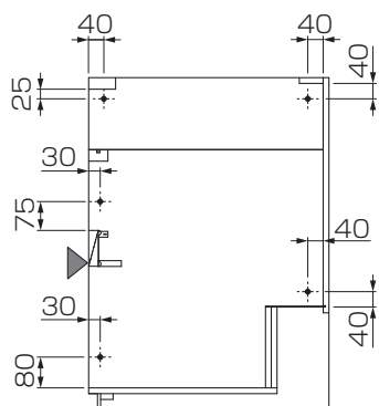
＜コンロ下ベースキャビネット 側面図＞
