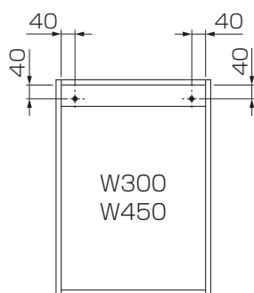
＜調理下ベースキャビネット 上面図＞
