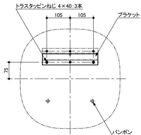
ブラケット取付位置
