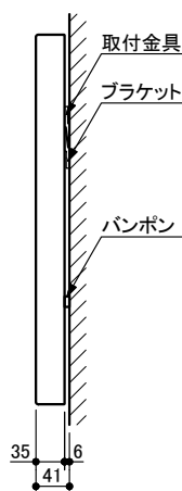
A-A' 断面図
