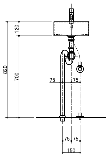
单水栓
