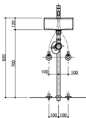
混合水栓
